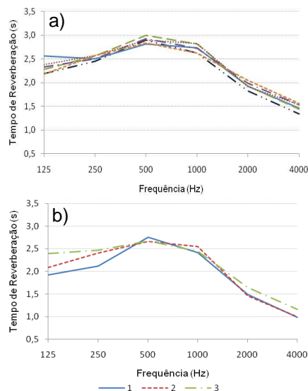
Quadro 1 – Valores dos Tempos de Reverberação médios medidos nas salas de culto principal e das mulheres.
