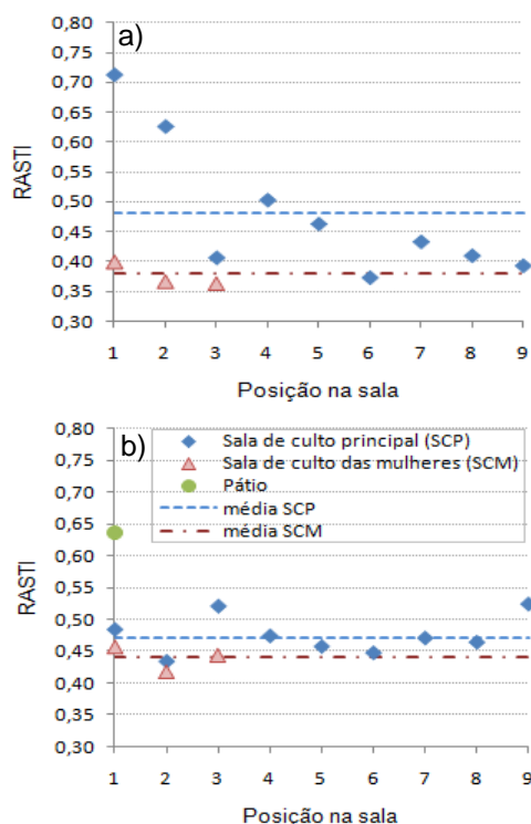
Figura 6 – Valores do RASTI obtidos para as várias posições na sala de culto principal e das mulheres com o Sistema de Reforço Electroacústico (SRS) desligado (a) e com este ligado no pátio e nas salas de culto (b).
