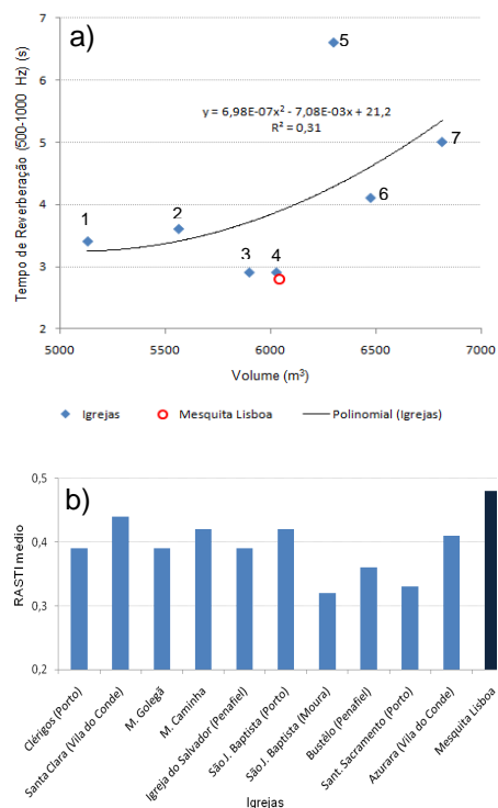
Figura 9 – a) Valores de TR em função do Volume das igrejas com volumes entre 5100 e 7300 m 3 e função de regressão; b) RASTI médio nas diversas igrejas e Mesquita de Lisboa.
