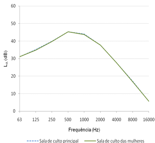
Figura 7 – Níveis sonoros médios nas salas de culto principal e das mulheres.
