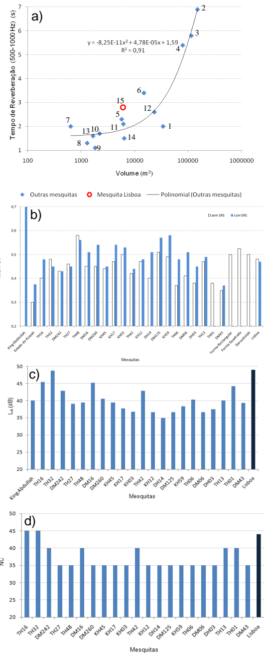
Figura 8 – Comparação entre mesquitas: a) Valores de TR em função do Volume com a respectiva função de regressão; b) RASTI médio; c) Níveis sonoros existentes; d) Níveis NC.
