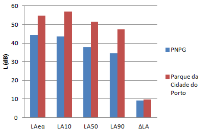
Figura 10 – Valores dos vários parâmetros acústicos nas áreas em comparação: Parque da Cidade (Porto) [4] e PNPG.
