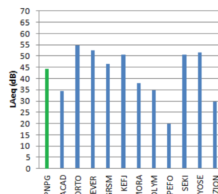
Figuras 8 (esq.) e 9 (dir.) - Comparação dos valores de L_{A10} e L_{Aeq} no PNPg e em parques dos EUA [3].
