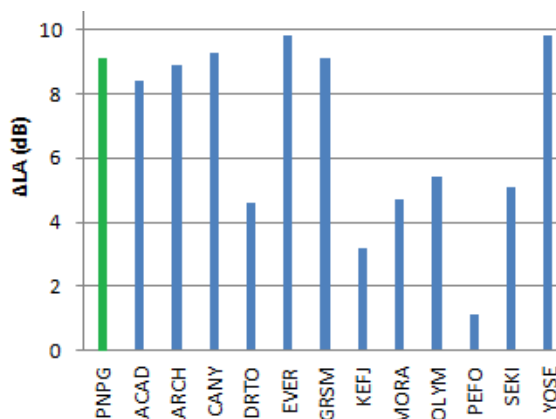
Figura 3 - Comparação dos valores de \Delta L_A (= L A10 - L A90 ) PNPG e em 12 parques dos EUA [3].
