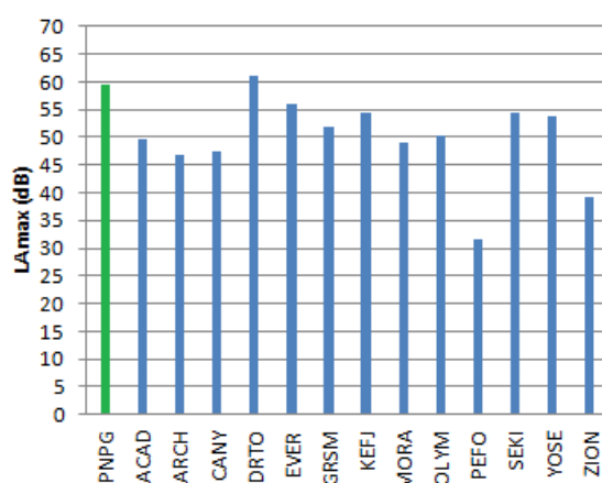
Figuras 4 (esq.) e 5 (dir.) - Comparação dos valores de L_{Amin} e L_{Amax} no PNPg com parques dos EUA [3].
