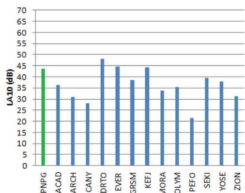
Figuras 8 (esq.) e 9 (dir.) - Comparação dos valores de L_{A10} e L_{Aeq} no PNPg e em parques dos EUA [3].
